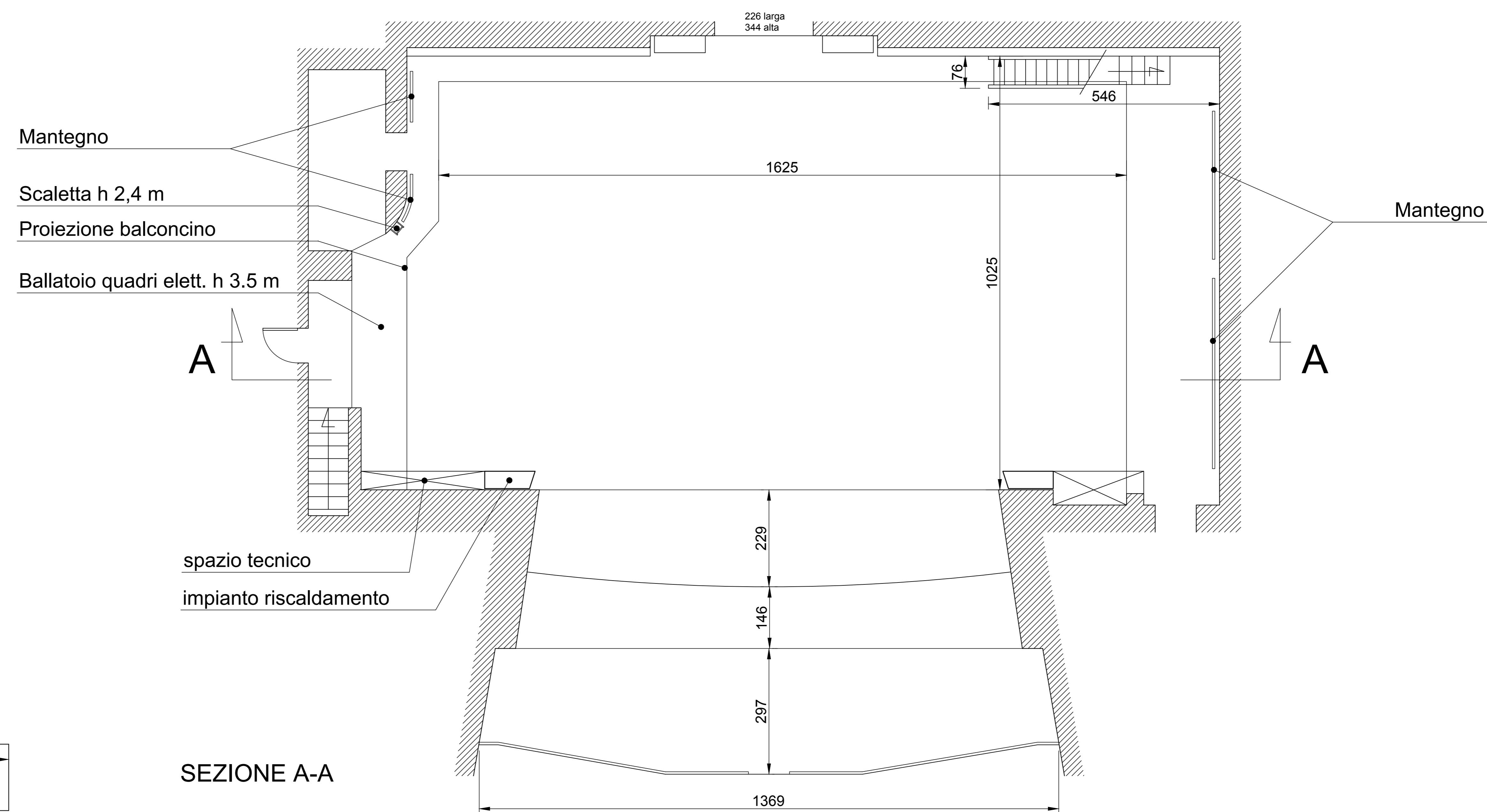
Dettaglio palco con buca d'orchestra chiusa 1:200
