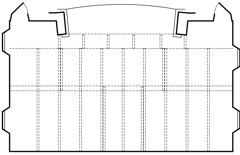
Pianta orditura primaria graticola
