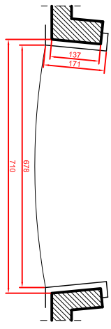
dettaglio pianta boccascena
