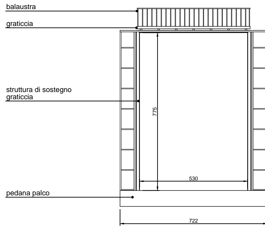
PROSPETTO STRUTTURA PALCO E GRATICCIA
