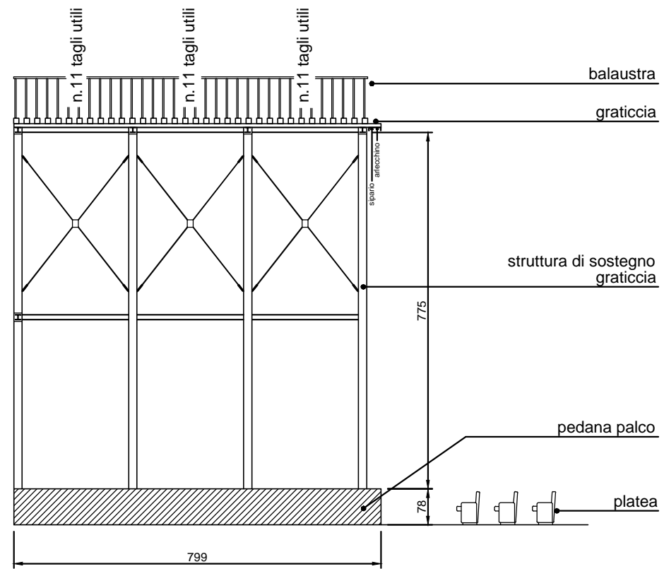
SEZIONE STRUTTURA PALCO E GRATICCIA
