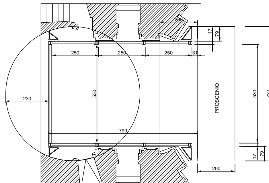
PIANTA POSIZIONAMENTO STRUTTURA PALCO E GRATICCIA
